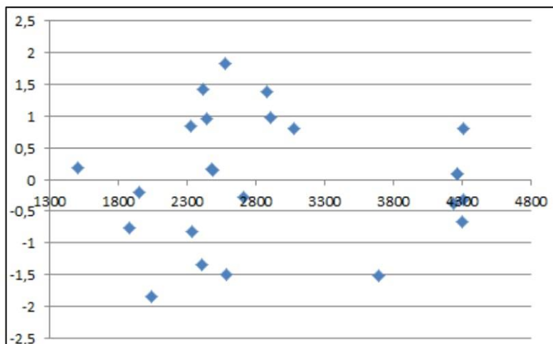
Figura 1 : Gráfico dos Resíduos Padronizados versus Preços Ajustados
