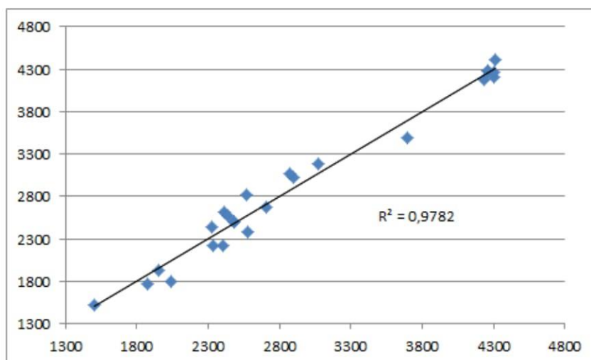
Figura 2: Preços Observados versus Preços Ajustados
